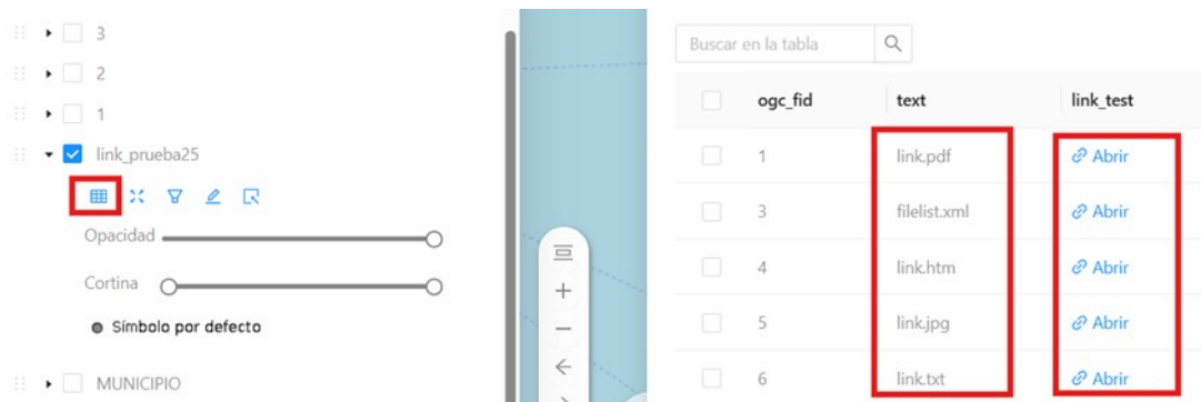
Figura 13. Campo enlace.
