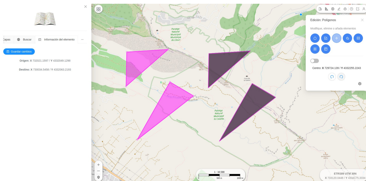
Figura 29. Trasladar geometría
