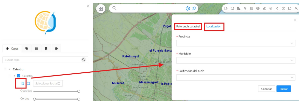
Figura 6. Búsqueda catastral
