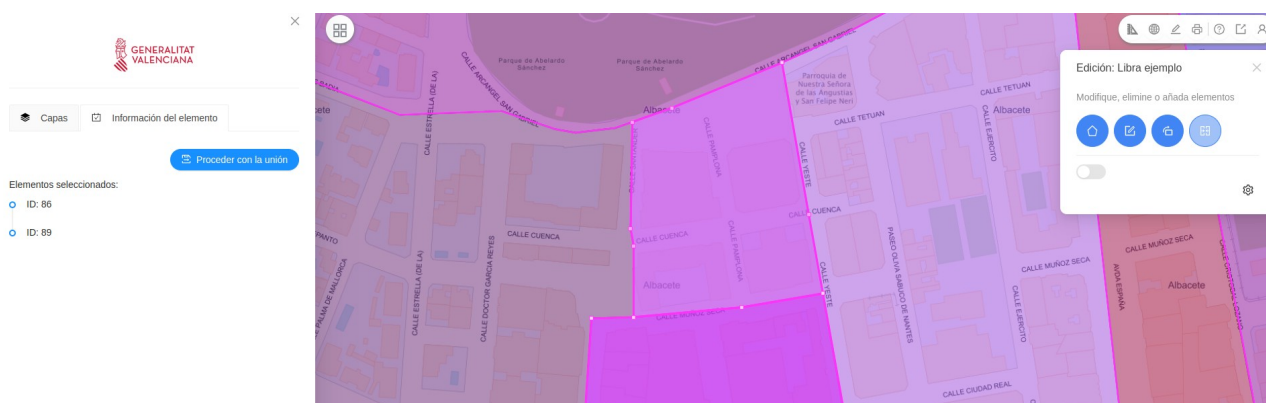
Figura 31. Unir geometrías
