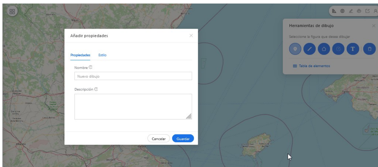
Figura 58. Añadir propiedades.
