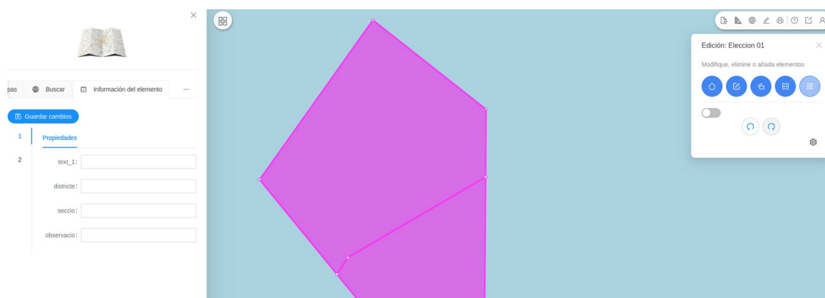
Figura 32. Dividir geometrías
