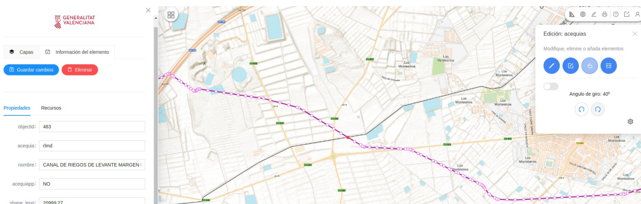
Figura 30. Girar geometría.
